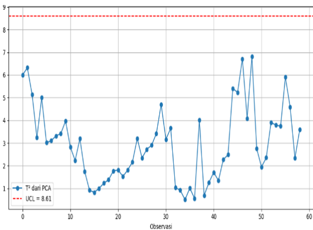
Gambar 5 Peta Kendali T^2 Hotelling (PCA)
