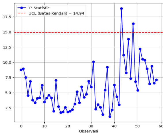
Gambar 4 Peta Kendali T^2 Hotelling klasik
