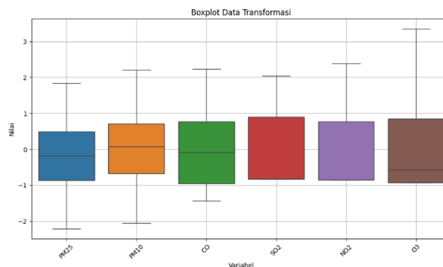
Gambar 2 Visualisasi Data pada Boxplot setelah Transformasi
