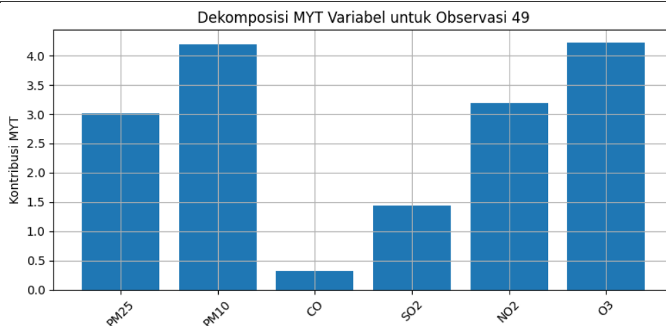
Gambar 7 Visualisasi hasil Dekomposisi MYT pada 19 Mei
