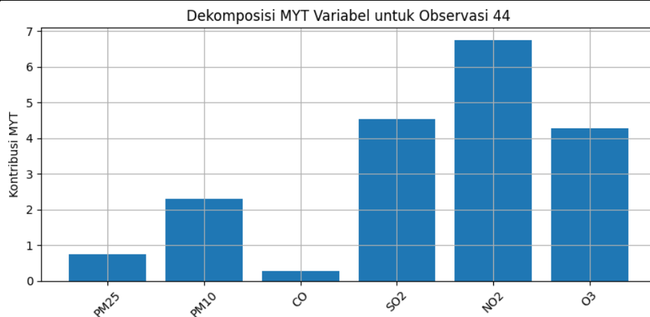
Gambar 6 Visualisasi hasil Dekomposisi MYT pada 14 Mei
