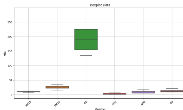
Gambar 1 Visualisasi Data pada Boxplot
